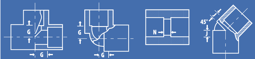
DIMENSIONES MÍNIMAS DEL CUERPO DE LAS CONEXIONES (ASTM D2846)
